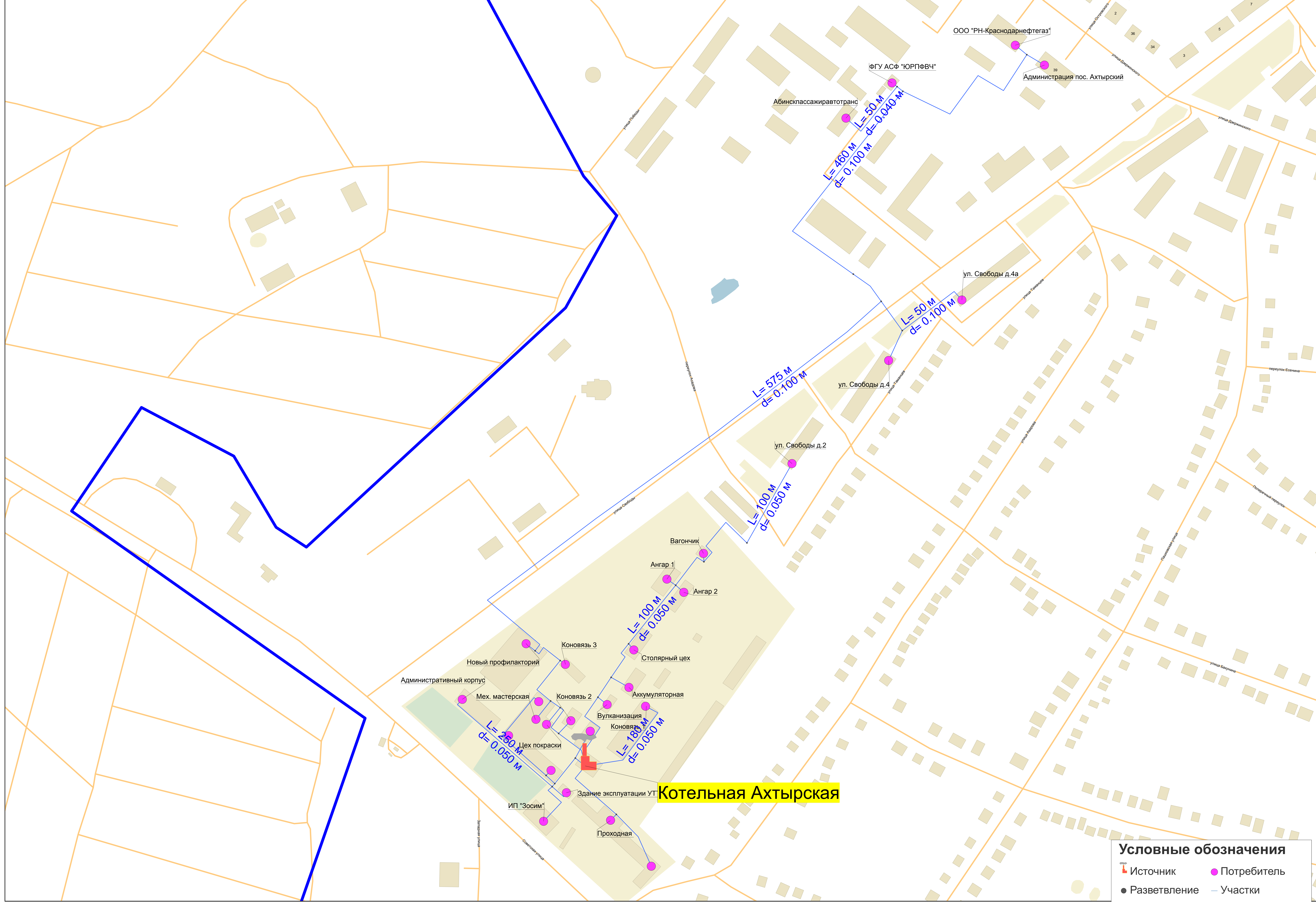
Рис. 4. Схема тепловых сетей котельной Ахтырская Ахтырского городского поселения
