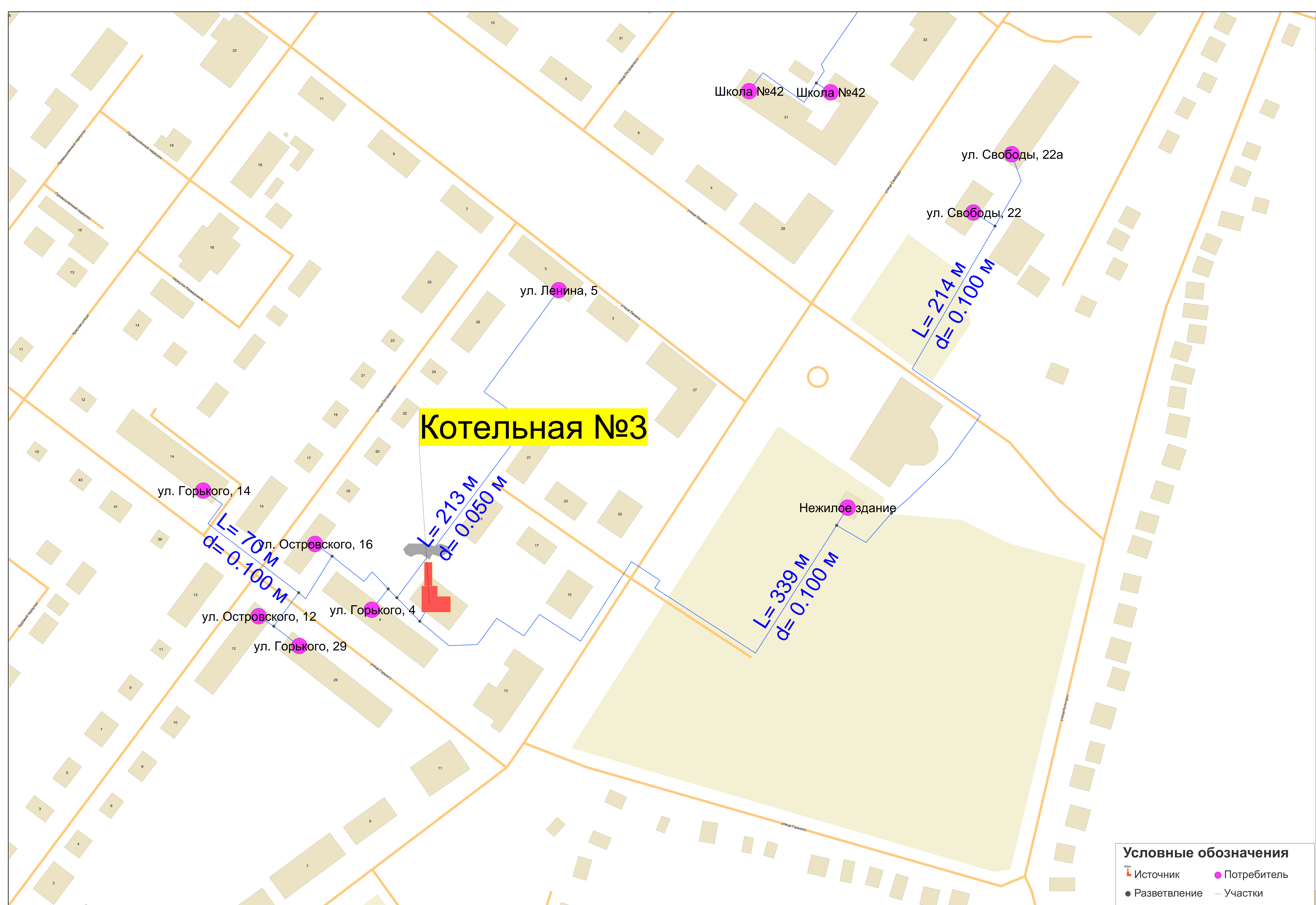
Рис. 2. Схема тепловых сетей котельной №3 Ахтырского городского поселения
